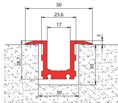
L-113 Canalina a terra alluminio Lavorazione pavimentazione Floor channel - Floor installation Bodenführung - Bodenvorbereitung
